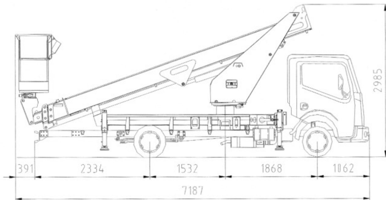
Figur 3: Aufbau der Arbeitsbühne PLA212 auf Nissan Cabstar F24.35/3 (cod.K.173.0.0.0.0)
