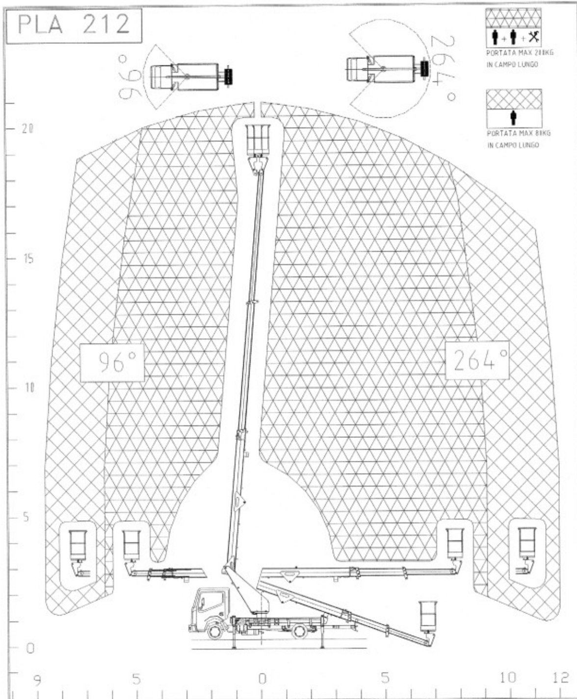
Figur 1: Arbeitsdiagramm langes Feld (cod. D.173.1.0.0.0)
