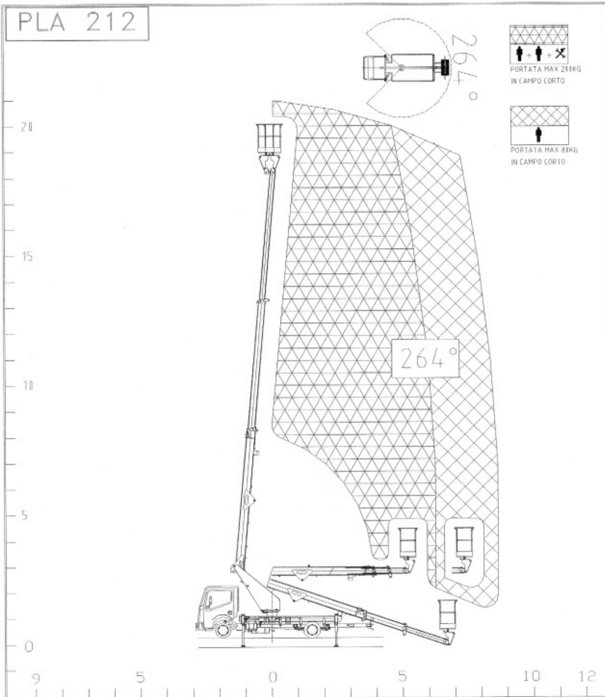
Figur 2 – Arbeitsdiagramm kurzes Feld (cod. D.173.2.0.0.0)
